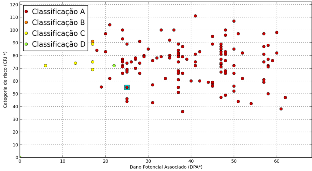
Figura 7 – CRI* e DPA* de todas as barragens na situação atual e após a implementação de todas as medidas propostas
